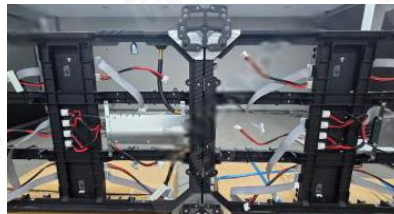
2. 캐비넷 사전조립
